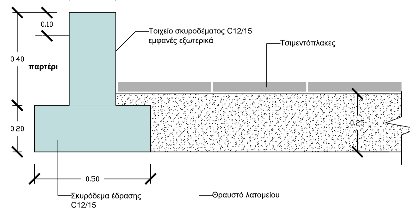
ΤΟΜΗ ΠΑΡΤΕΡΙΟΥ ΑΠΟ ΤΟΙΧΕΙΟ ΒΕΤΟΝ ΚΛ 1:10
