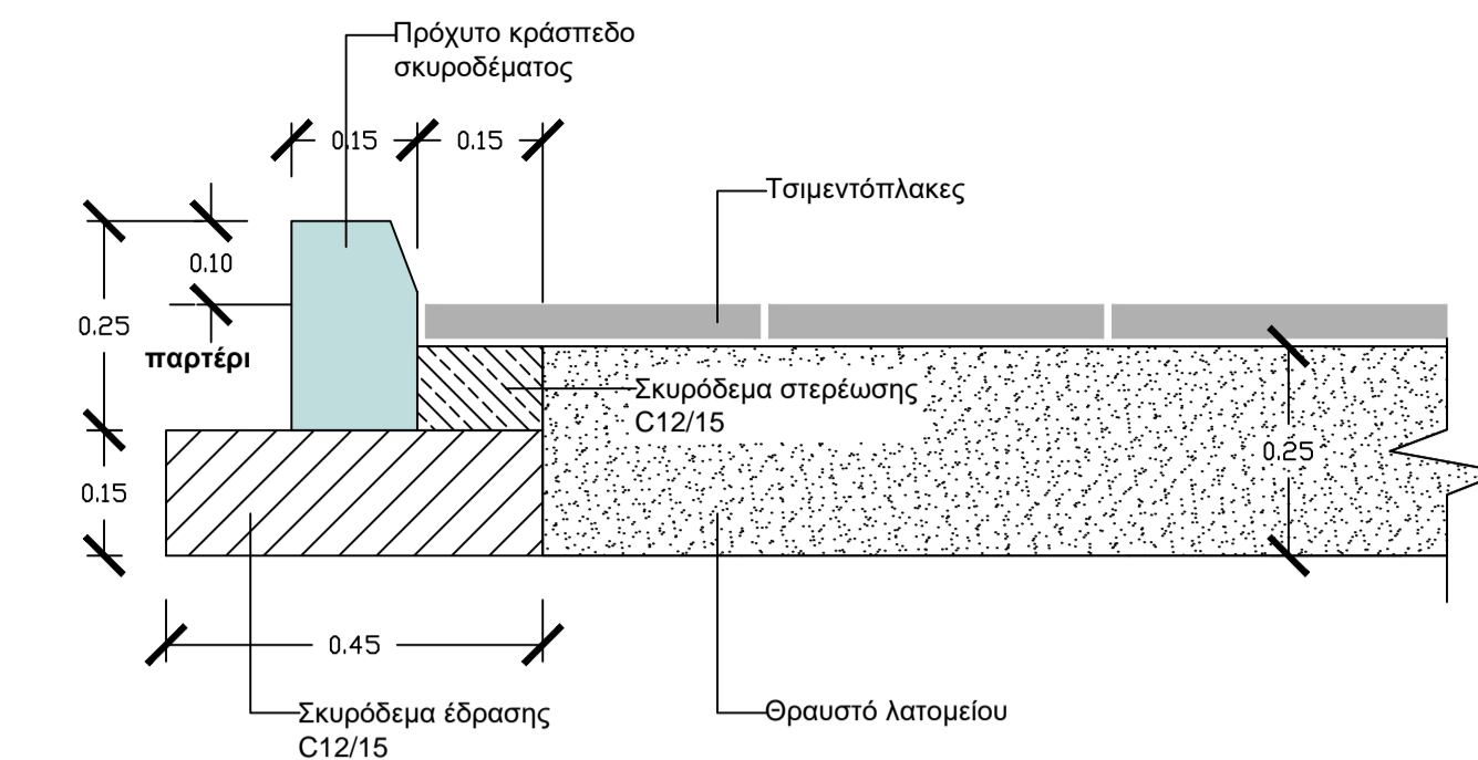
ΤΟΜΗ ΠΑΡΤΕΡΙΟΥ ΑΠΟ ΤΟΙΧΕΙΟ ΒΕΤΟΝ ΚΛ 1:10
