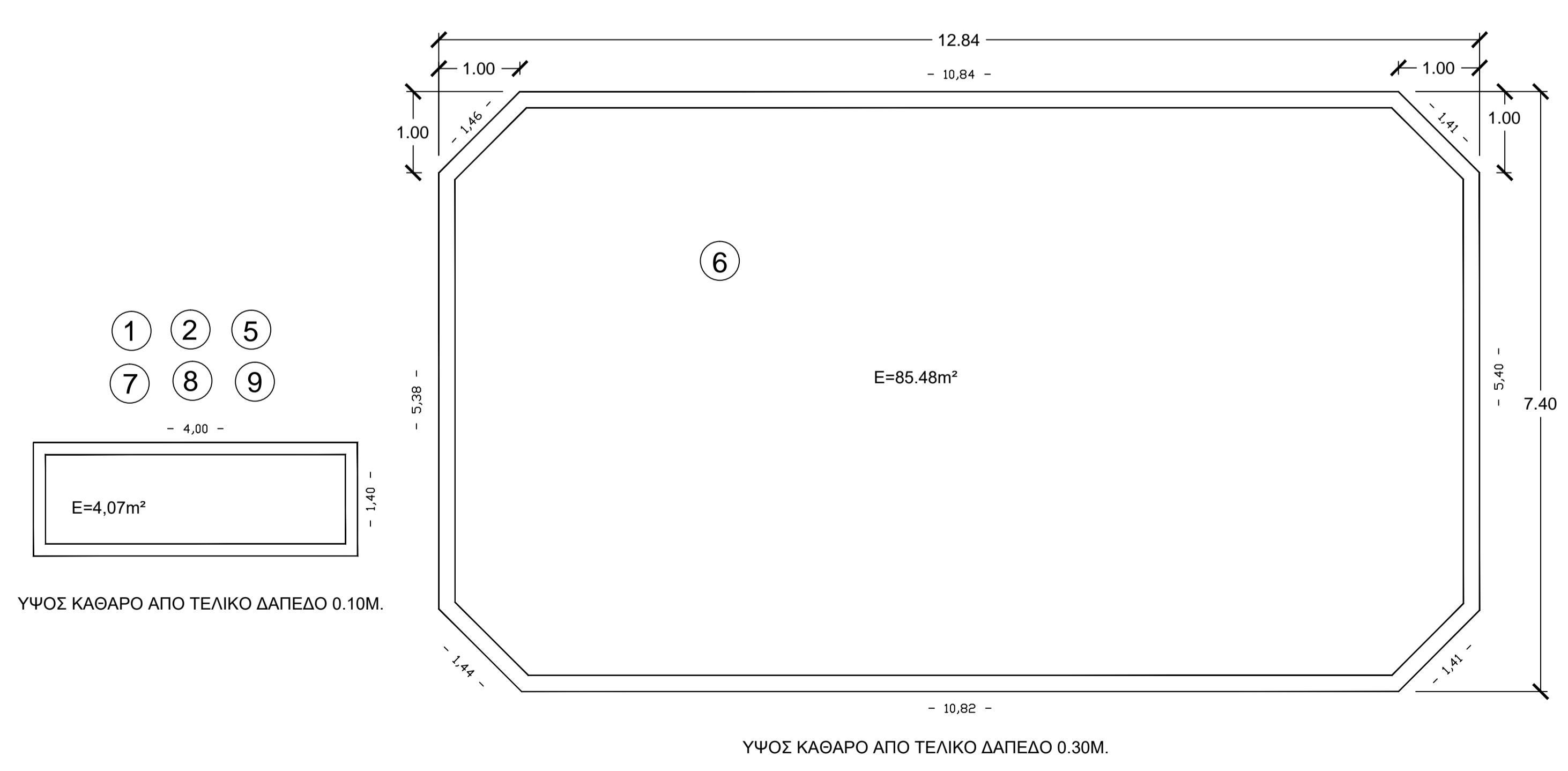
ΛΕΠΤΟΜΕΡΕΙΕΣ ΠΑΡΤΕΡΙΩΝ 02 ΚΛ. 1:50
