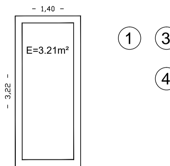
ΛΕΠΤΟΜΕΡΕΙΕΣ ΠΑΡΤΕΡΙΩΝ 01 ΚΛ. 1:50
