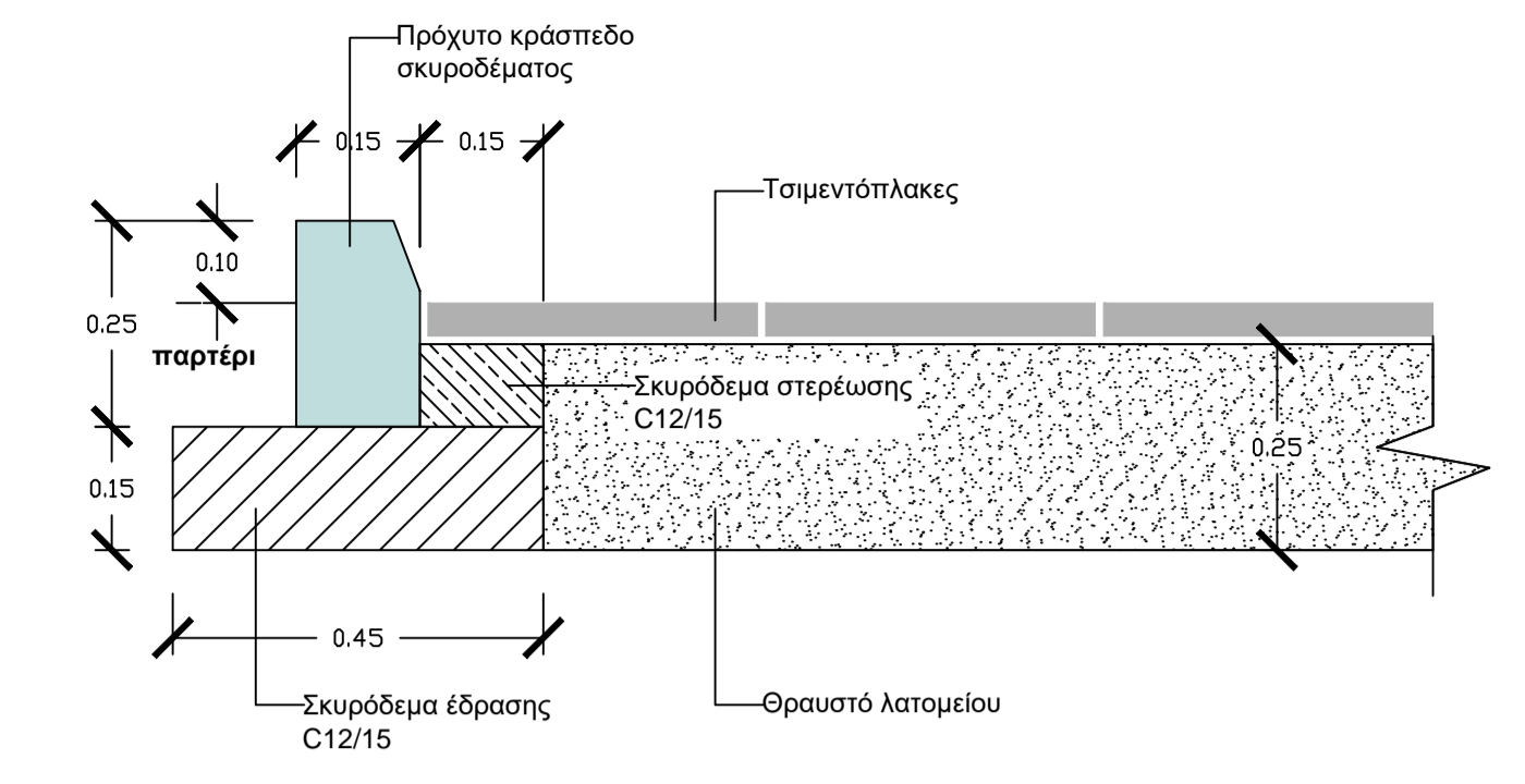
ΤΟΜΗ ΠΑΡΤΕΡΙΟΥ ΑΠΟ ΤΟΙΧΕΙΟ ΒΕΤΟΝ ΚΛ 1:10
