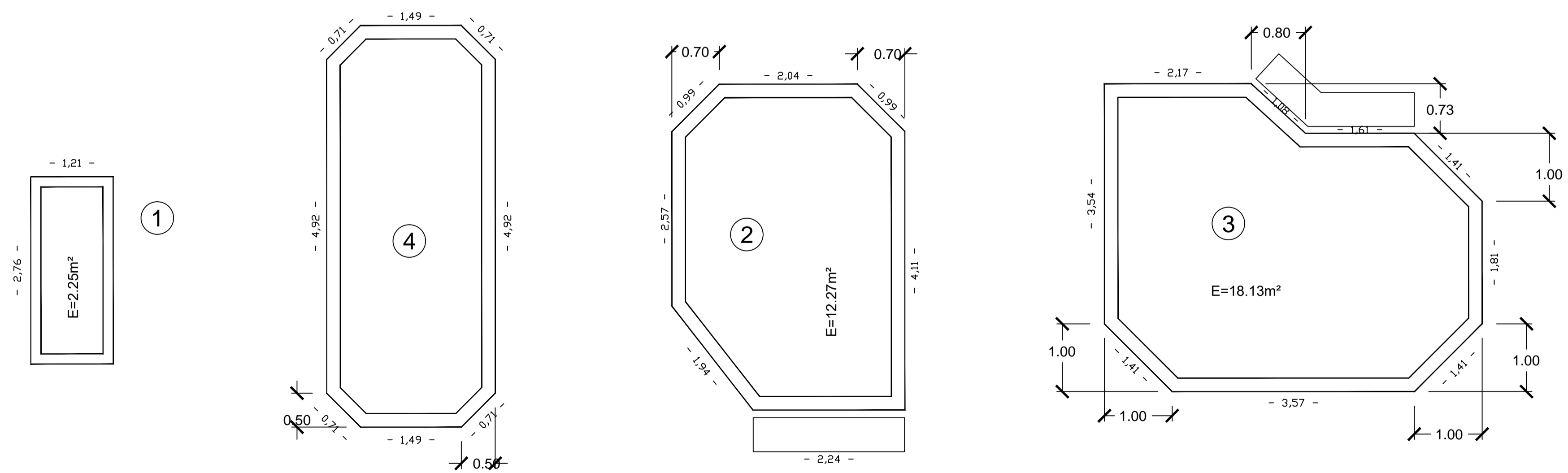
ΛΕΠΤΟΜΕΡΕΙΕΣ ΠΑΡΤΕΡΙΩΝ 10 ΚΛ. 1:50
