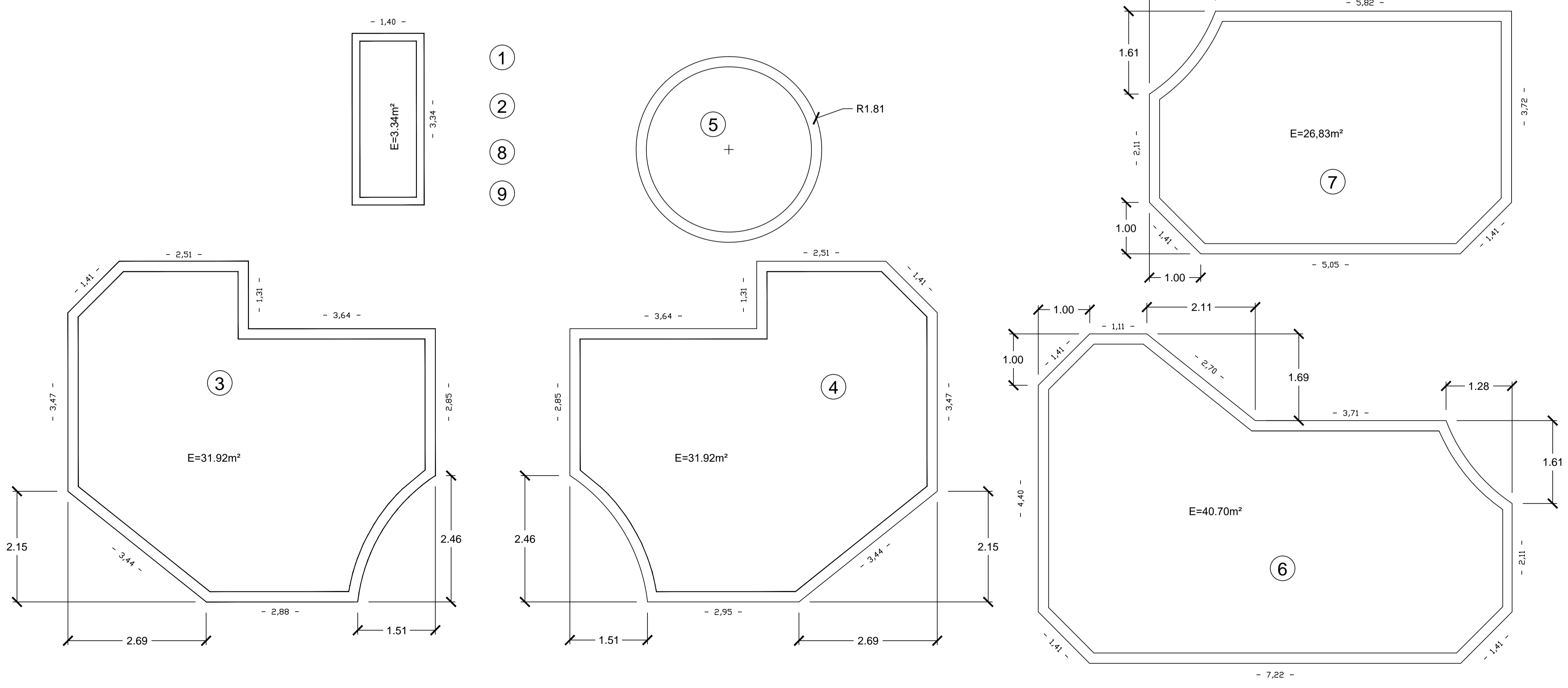
ΛΕΠΤΟΜΕΡΕΙΕΣ ΠΑΡΤΕΡΙΩΝ 04 ΚΛ. 1:50
