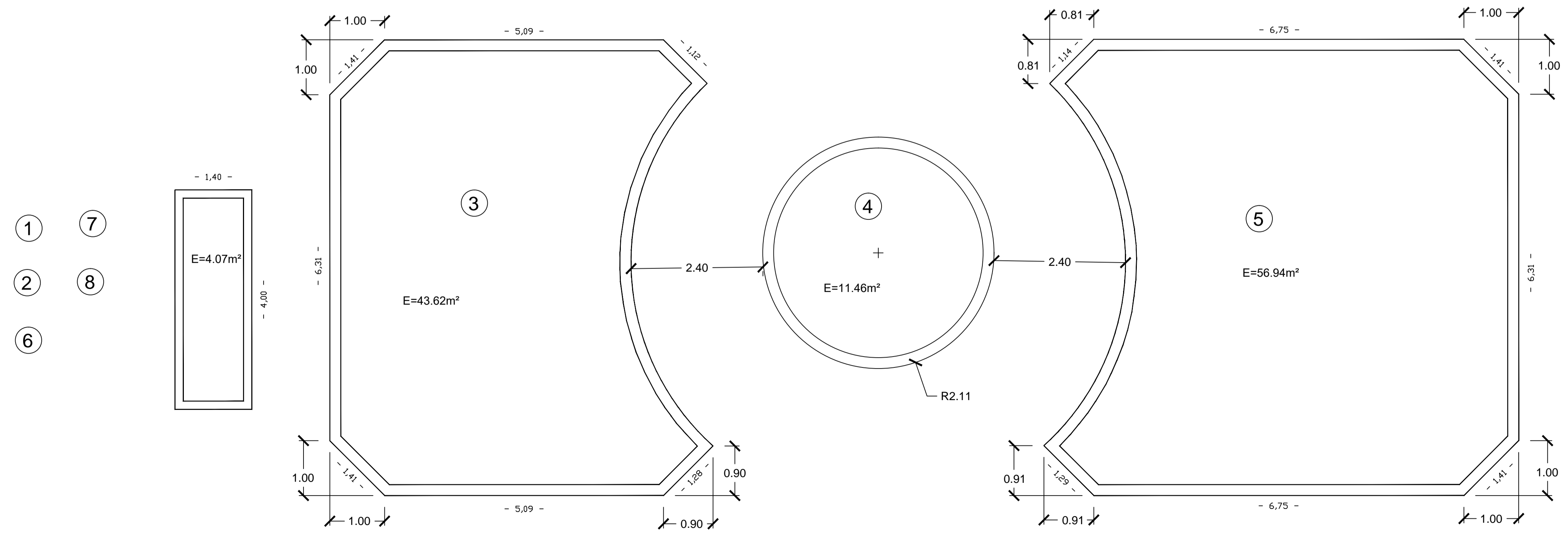
ΛΕΠΤΟΜΕΡΕΙΕΣ ΠΑΡΤΕΡΙΩΝ 06 ΚΛ. 1:50
