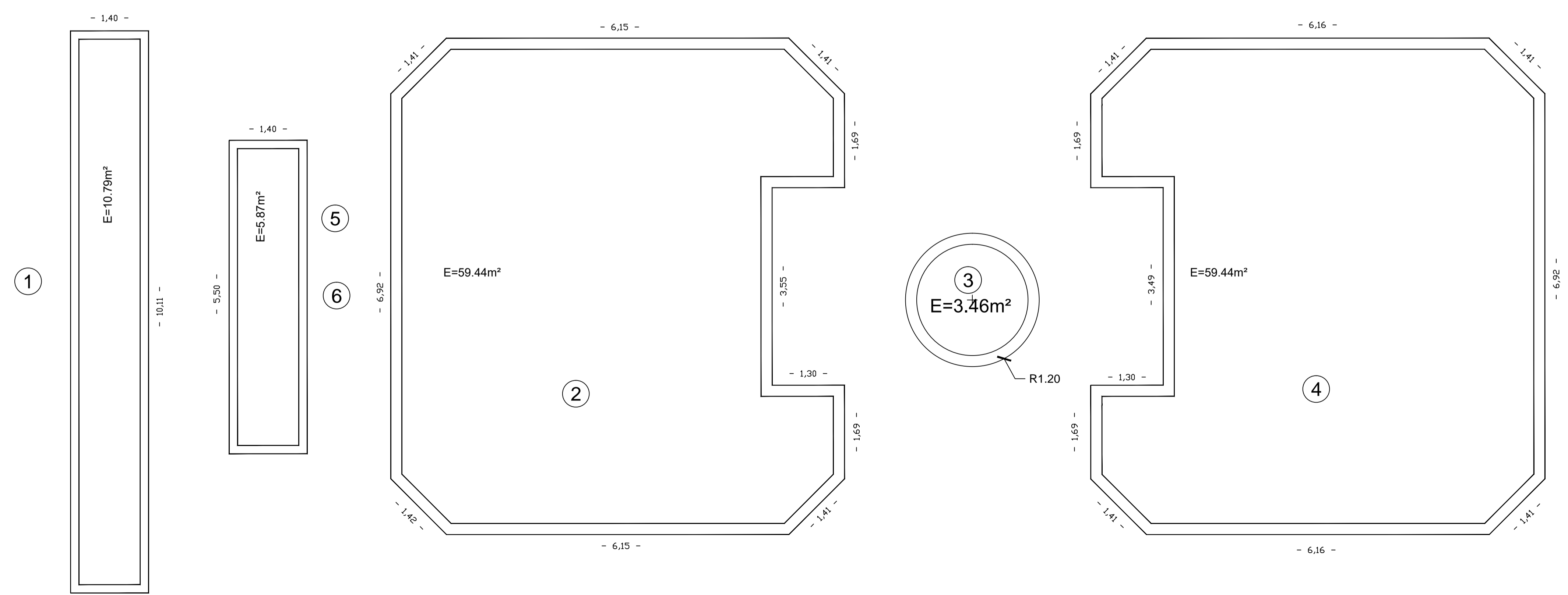
ΛΕΠΤΟΜΕΡΕΙΕΣ ΠΑΡΤΕΡΙΩΝ 11 ΚΛ. 1:50
